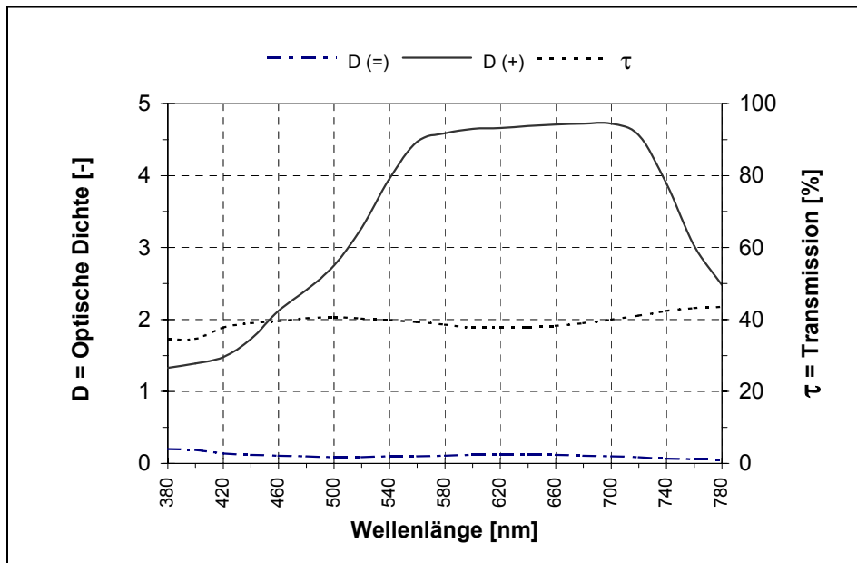
D(+) Dichte in Sperrrichtung, D(-) - in Durchlaßrichtung bei 100% polarisiertem Prüflicht
