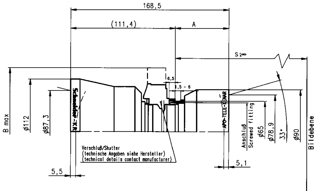
APO-TELE-XENAR 9,0/600 in Verschluß 3 Shutter 3
